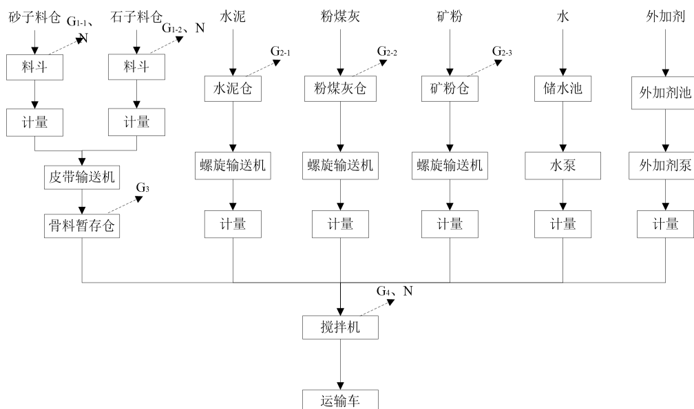
图 2-4 混凝土生产工艺及产污环节图
