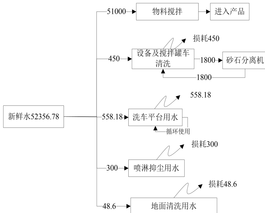
图 2-3 本项目水平衡图 ( \text{m}^3/\text{a} )
