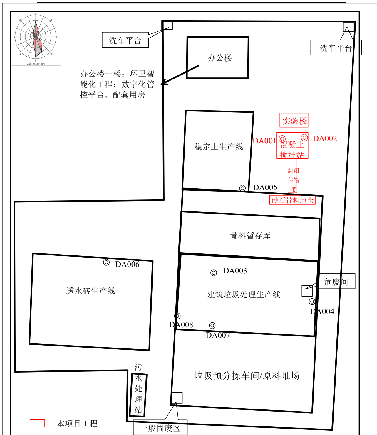
图 2-2 平面布置图
